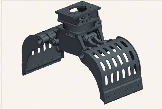
MG-450 · EXTERIOR VIEW · RAL 7026
