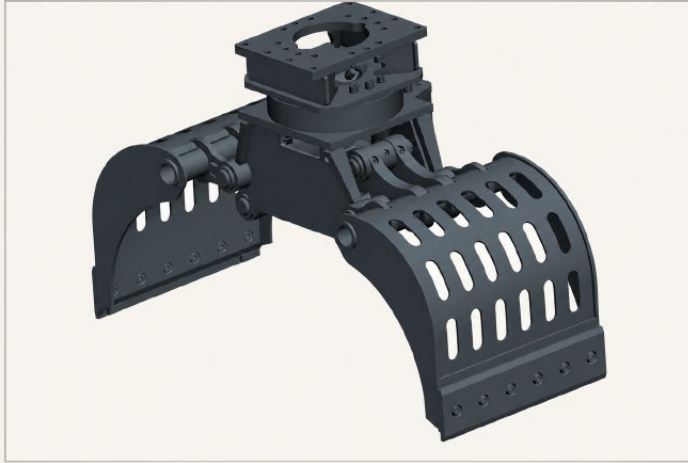
MG-400 · EXTERIOR VIEW · RAL 7026
