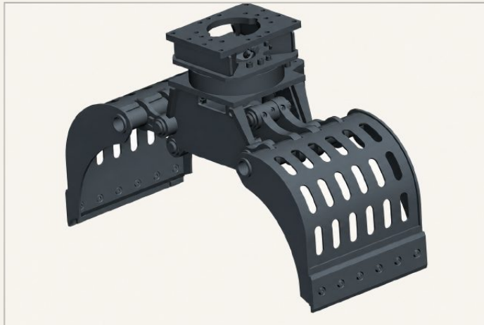
FIG. 01 · MG-150 · VISTA EXTERIOR · RAL 7026
