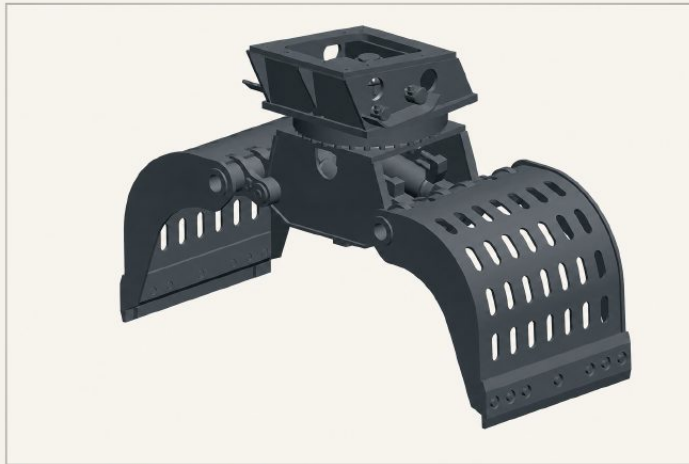
MG-1400 · EXTERIOR VIEW · RAL 7026
