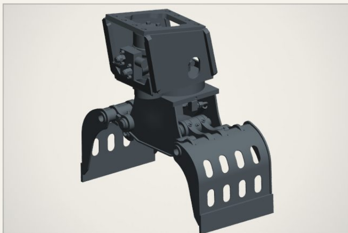
MG-100 · EXTERIOR VIEW · RAL 7026
